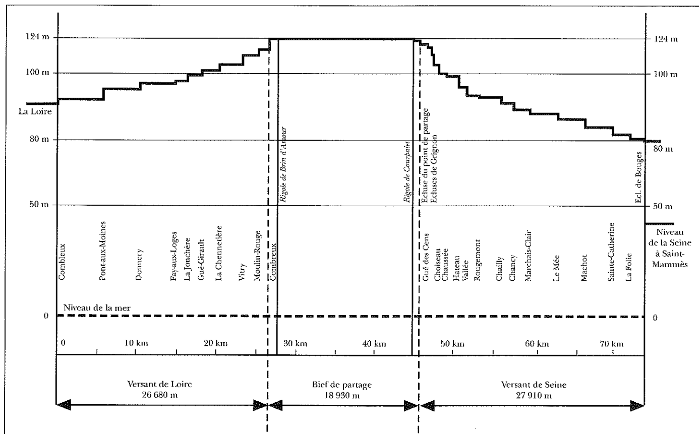
Profil général du canal d'Orléans.
